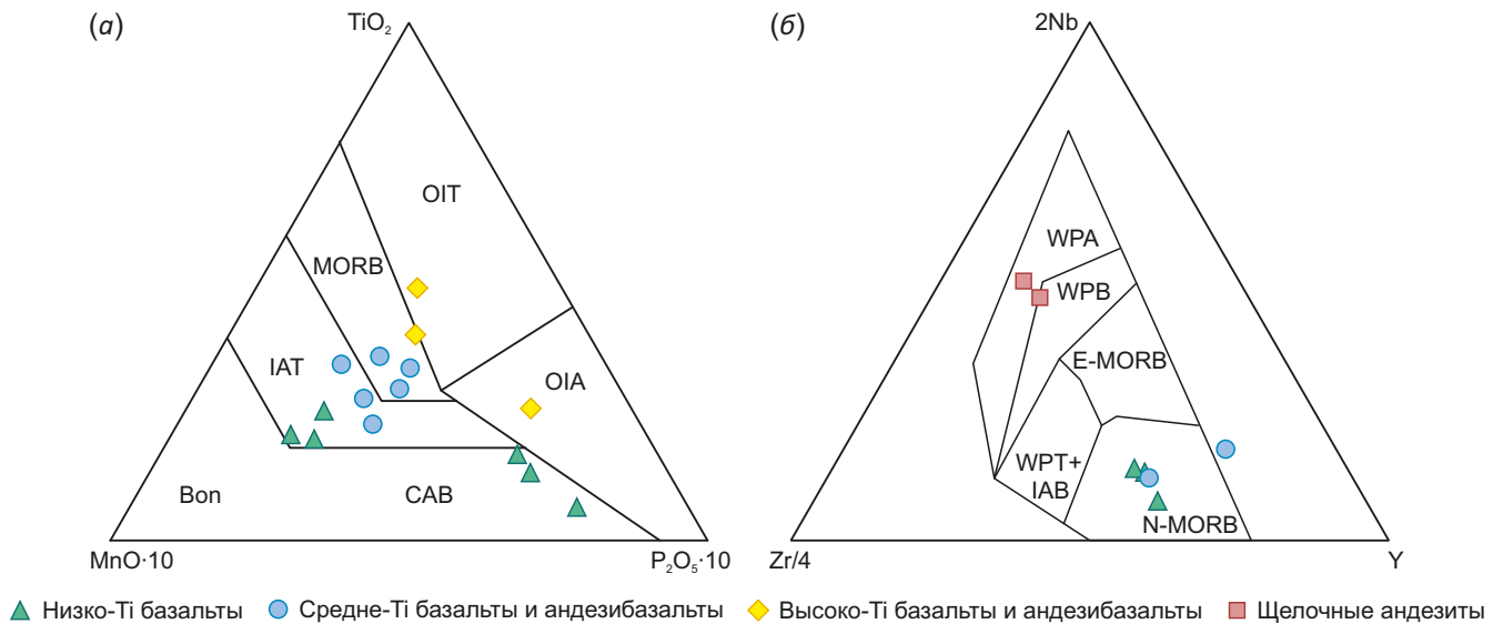
Рис. 9. Тектонические дискриминационные диаграммы. (а) – диаграмма MnO - TiO_2 - P_2O_5 [Mullen, 1983]; (б) – диаграмма Zr/4 - 2Nb - Y [Meschede, 1986]; WPA – внутриплитные щелочные базальты, WPB – внутриплитные базальты, WPT+IAB – внутриплитные толеиты и островодужные базальты, Bon – бониниты, OIT – толеиты океанических островов/симаунтов, OIA – щелочные базальты океанических островов, IAT – островодужные толеиты, CAB – известково-щелочные базальты, MORB – базальты срединно-океанических хребтов.
