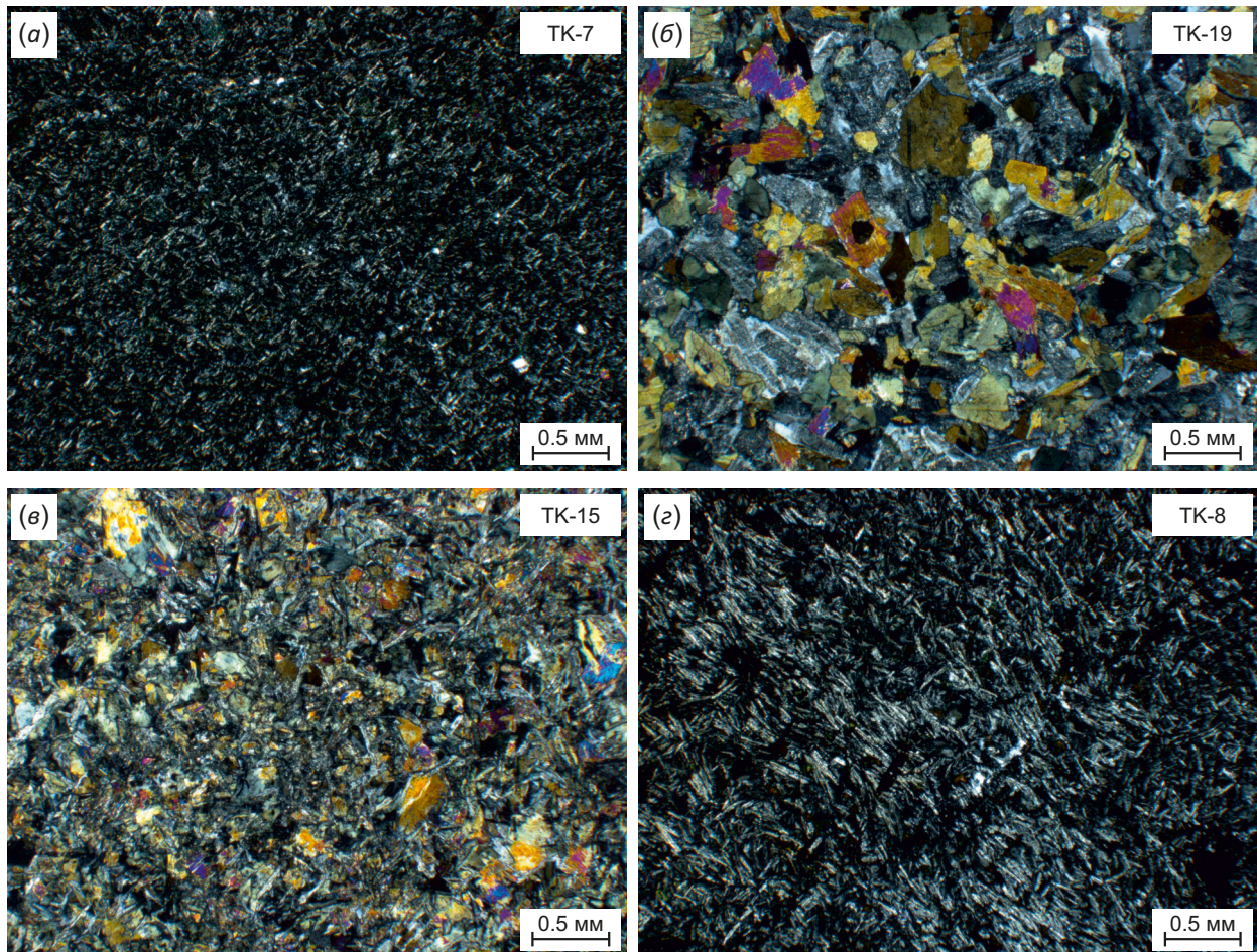
Рис. 5. Фото шлифов магматических пород ТАК. (а) – афировый базальт; (б) – габбро; (в) – долерит; (г) – андезит.
