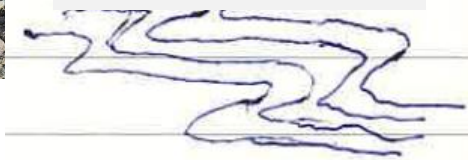
Шевронные складки
